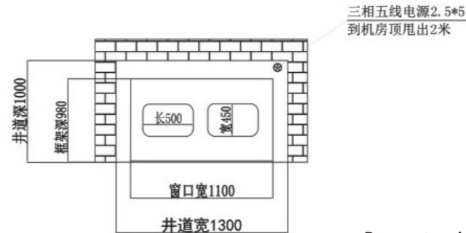
Parameter size of vegetable conveyor 传菜机参数尺寸
